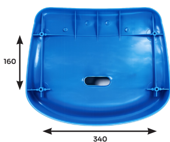
Otwory pod wkręt do drewna fi 6, głębokość otworów 25 mm.
